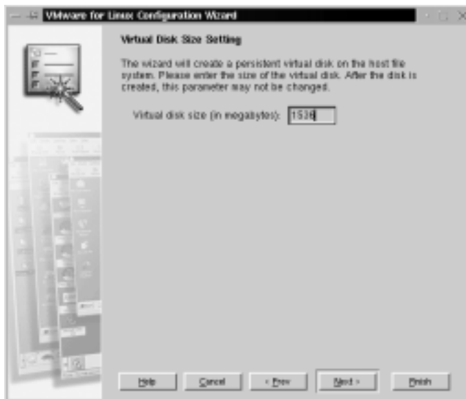
Abbildung 11.3: Größe der virtuellen Platte
