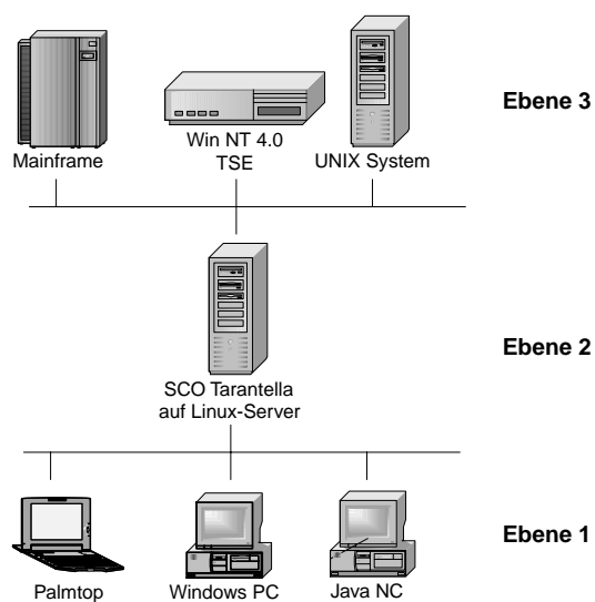
Abbildung 11.18: Die 3 Ebenen aus Tarantella-Sicht
